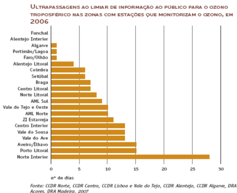
Figura 40 - Ultrapassagens ao limiar de informação ao público para o ozono troposférico nas zonas com estações que monitorizam o ozono, em 2006. Fonte: REA 2006
